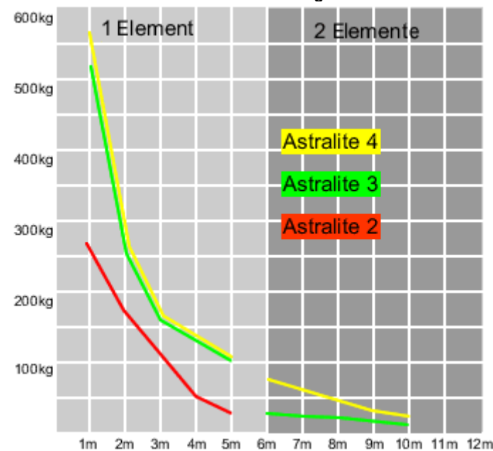
VERTEILTE LAST kg/m
